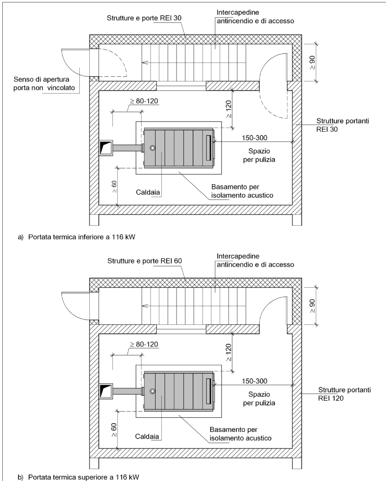
Figura 81.8 - Esempio di centrale termica alimentata a gas di rete con accesso da intercapedine antincendio di larghezza non inferiore a 0,90 m. Caratteristiche costruttive e distanze minime consigliate per gli spazi attorno al generatore
